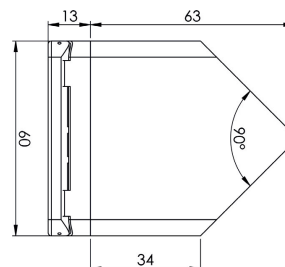
SIDE (LID)
